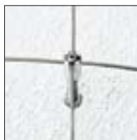
ASS Kreuzklemme 3 D mit Wandanschluß M 12
